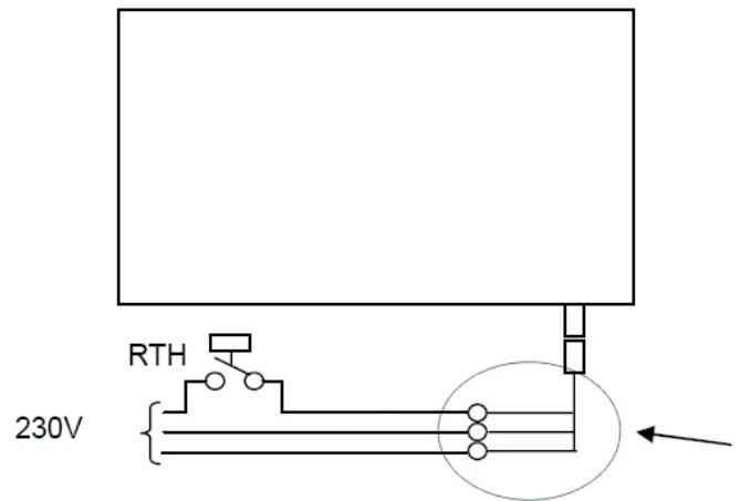
Figuur: Aansluitschema
